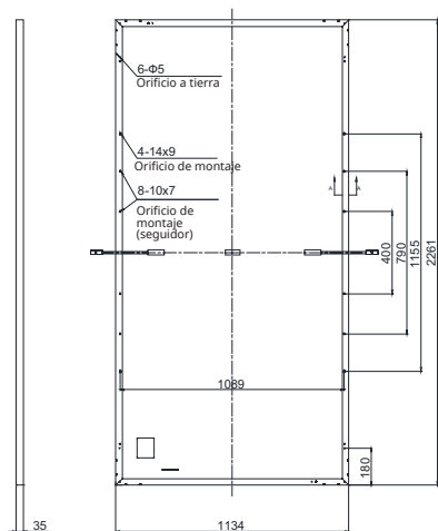
Vista trasera
